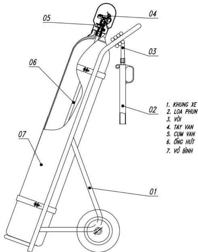
BÌNH CHỮA CHÁY XE ĐẨY CO2
